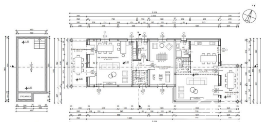
GRUNDRISS ERDGESCHOB
