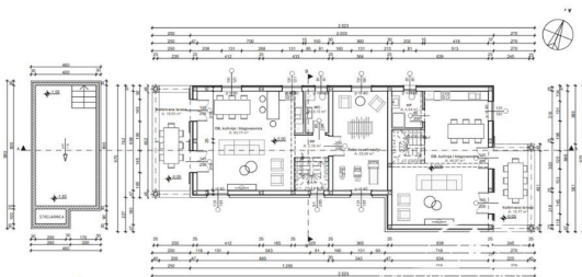
GRUNDRISS ERDGESCHOB
