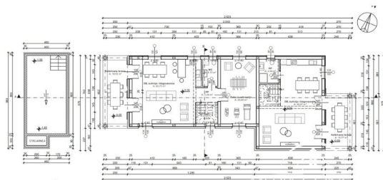
GRUNDRISS ERDGESCHOB
