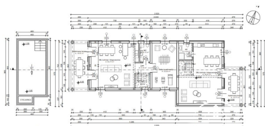
GRUNDRISS ERDGESCHOB
