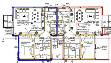
GRUNDRISS ERDGESCHOß
